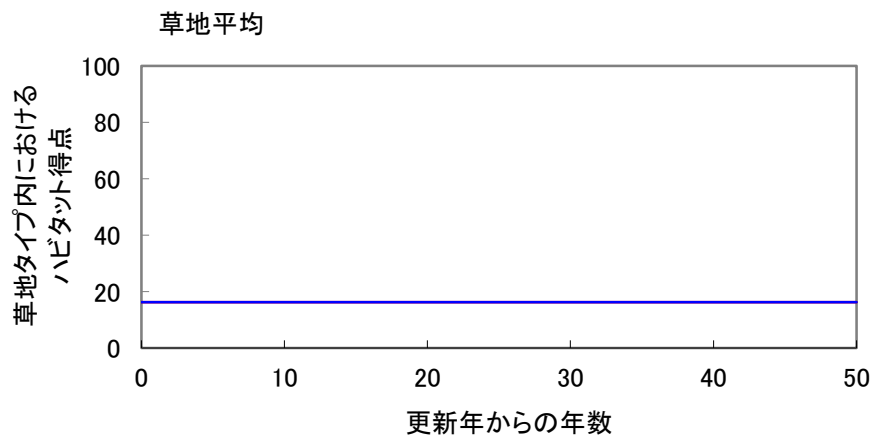
図. 環境タイプごとの評価基準値とハビタット得点の推移
